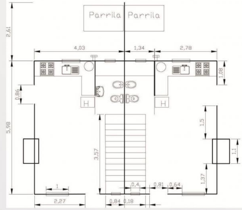
PLANTA ALTA
