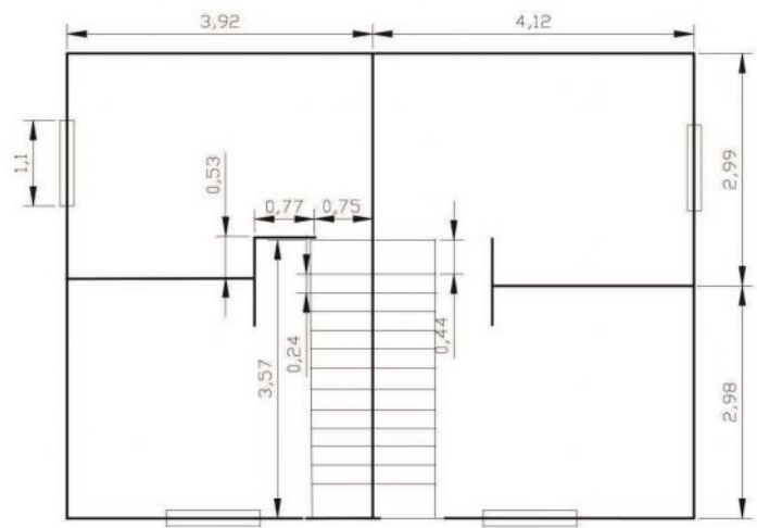
PLANTA ALTA
