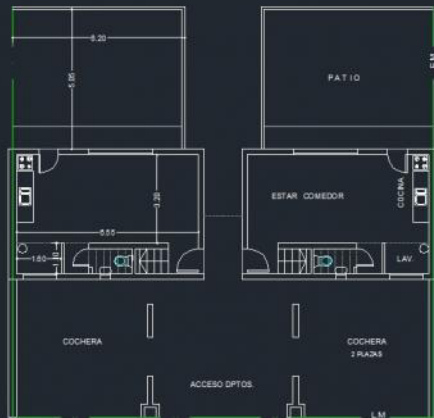
planta BAJA
